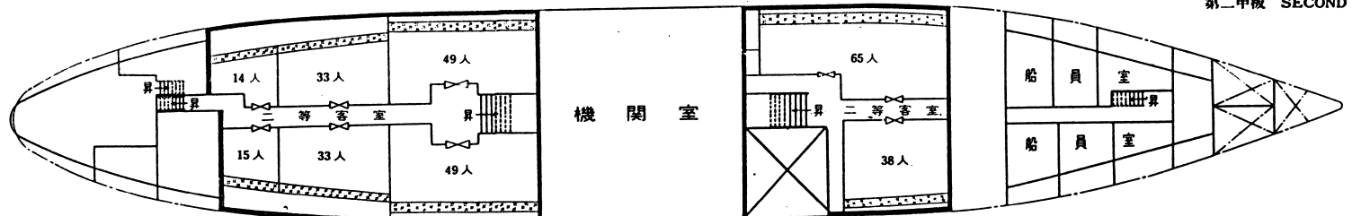
第二甲板 SECOND DECK
